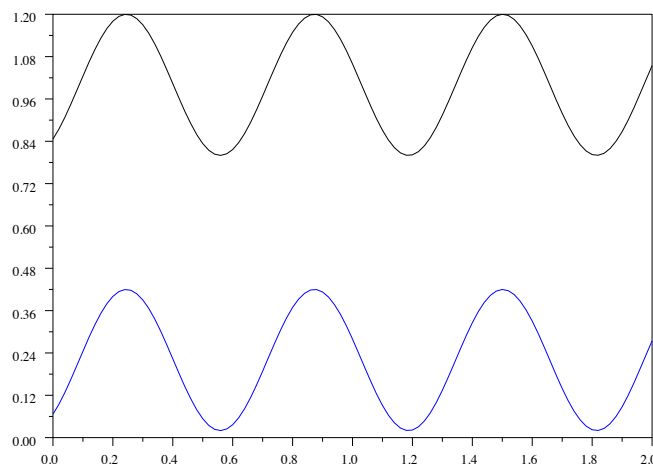
Cas linéaire : approximation du système (8), \Delta t = 0,02 .
